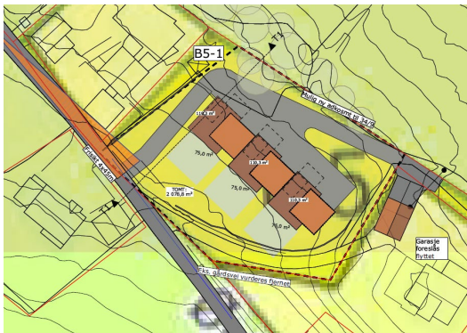
Figur 14 Situasjonsplan, foreløpig.
